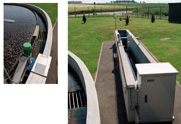
DEBITMETRE EAUX TRAITEES
